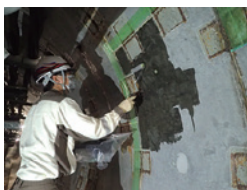
② プライマー塗布
