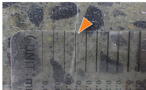
▲ひび割れの可視化(ひび割れが白く浮き出る)
