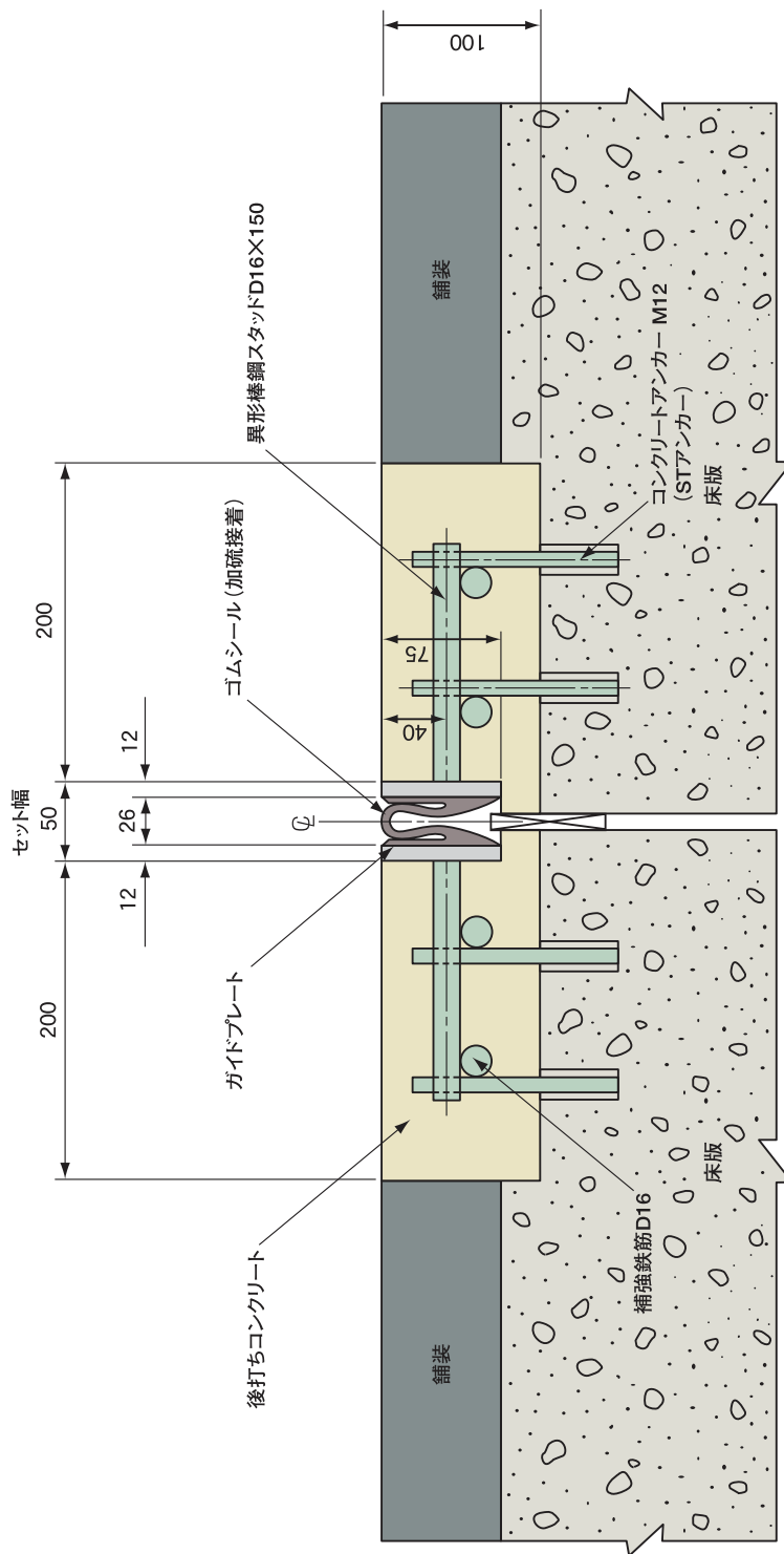
断面図
