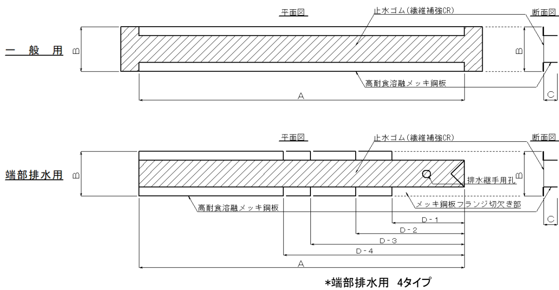
[クローザーSS 一般図]
