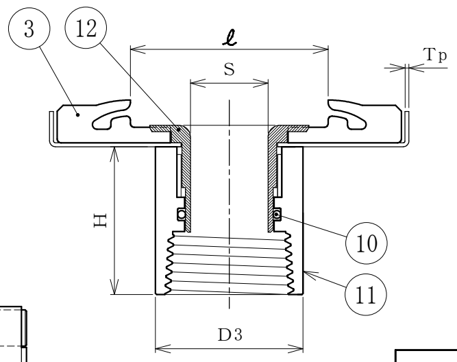
断面詳細図
