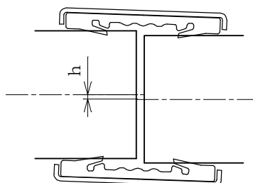
管中心線のズレ h
