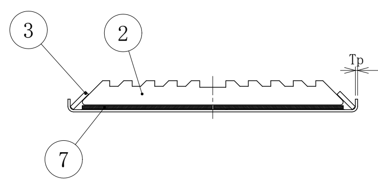
A-A断面詳細図
