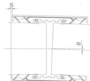
管中心線の曲がり \theta / カップリングの傾き S
