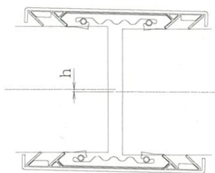
管中心線のズレ h
