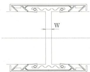
管と管の間隔 W
