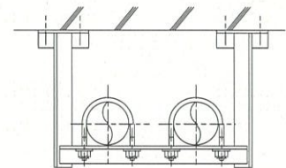
鋼棒吊り
