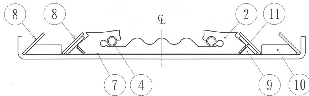
断面図
