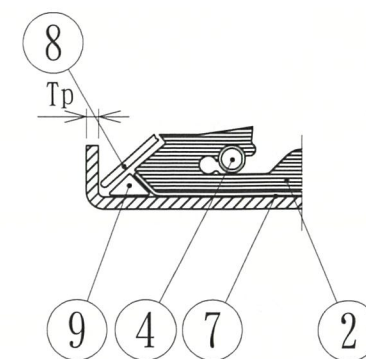
G-20~40E 断面図
