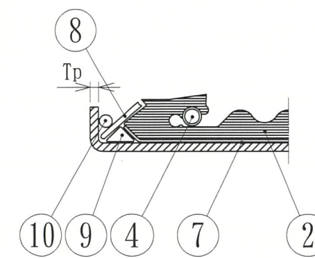
G-50~150E 断面図
