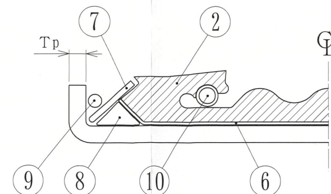
G-200E 断面図
