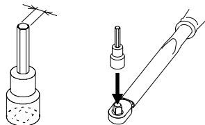
ソケットサイズ (二面幅)
