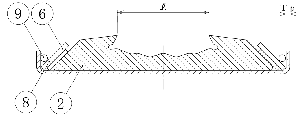
断面詳細図
