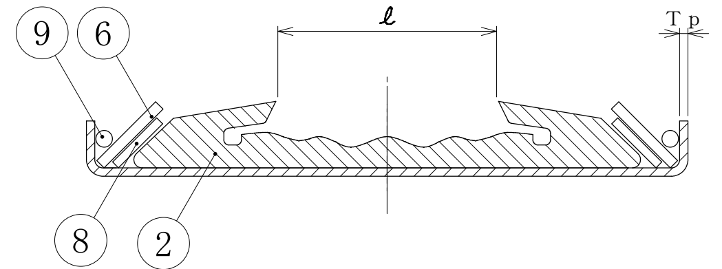
断面詳細図
