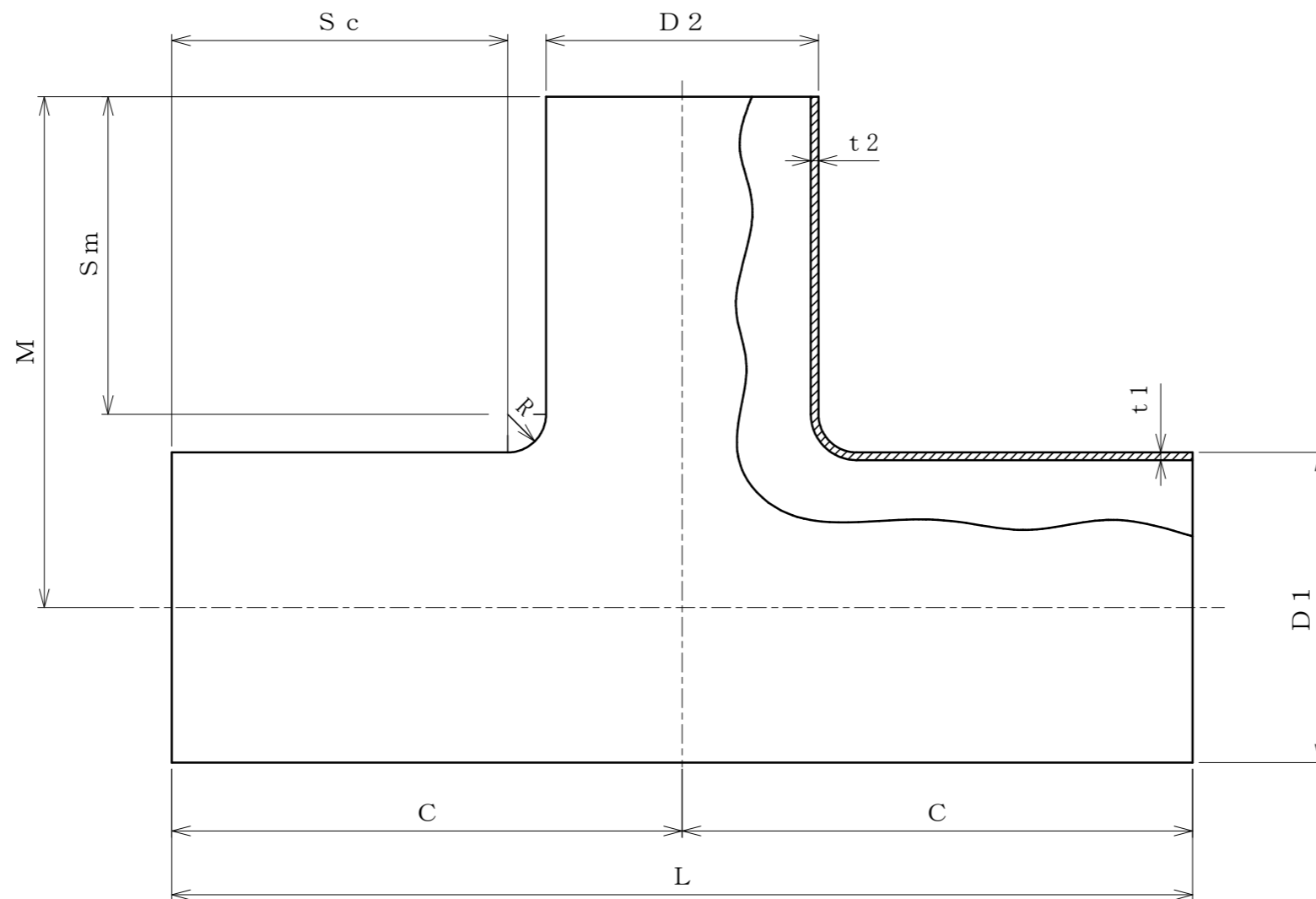
標準寸法
