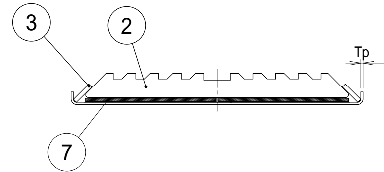
A - A 断面詳細図
