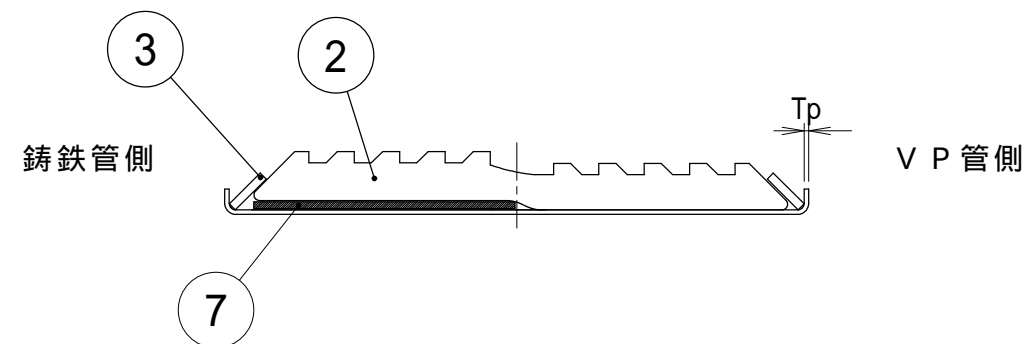
A - A 断面詳細図
